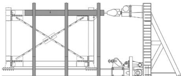
a. MRF specimens
