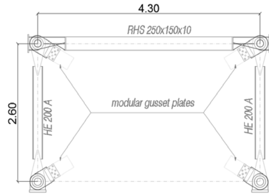
b. PC test frame
