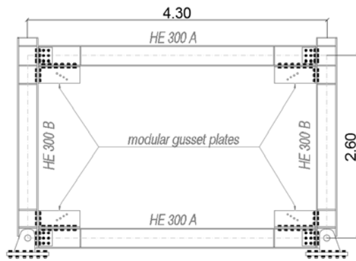
a. MRF test frame
